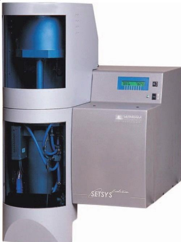
高溫腐蝕分析 儀 (TGA)
